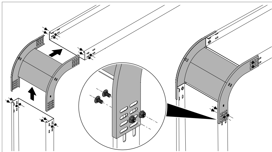
Slika 66: Montaža vertikalne krivine sa silaznim nagibom
