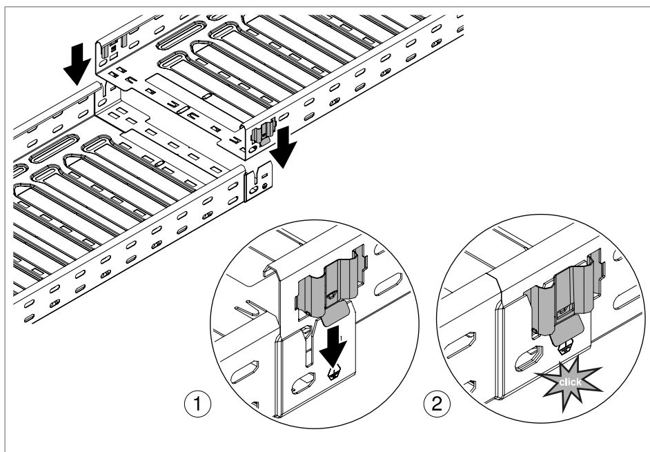
Slika 18: Uskočna spojica Magic sa opružnim elementom
