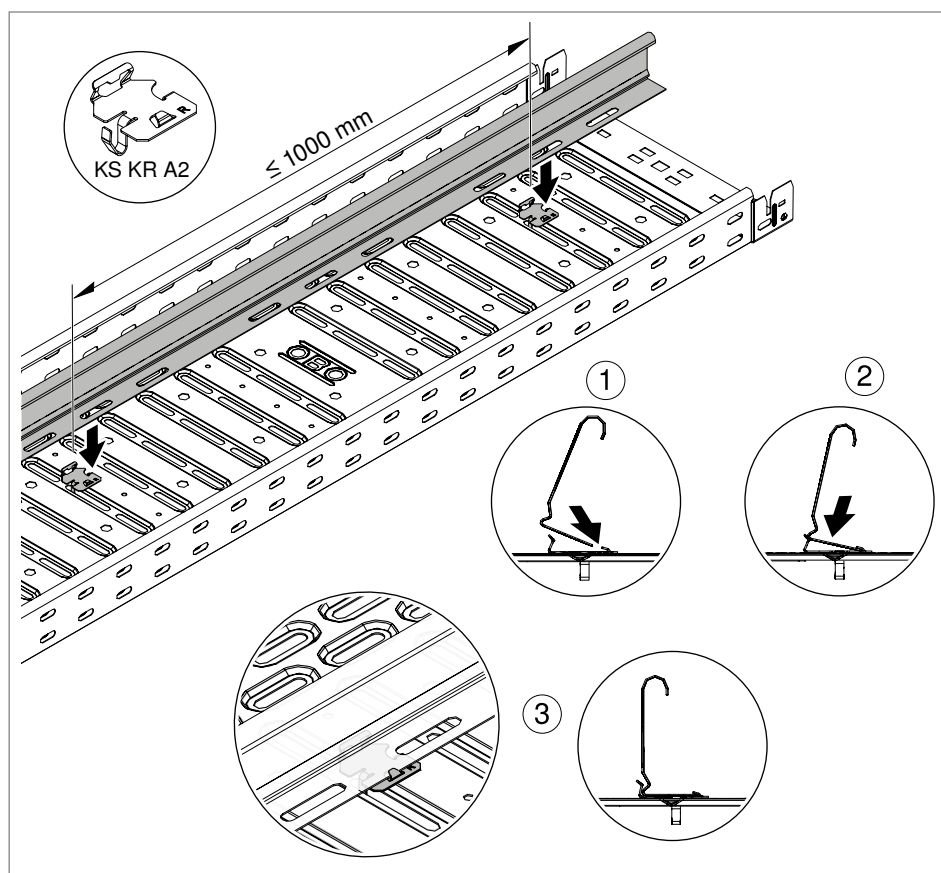
Slika 79: Postavljanje pregrade u stezni komad
