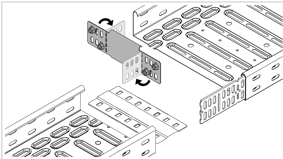
Slika 72: Savijanje reducira
