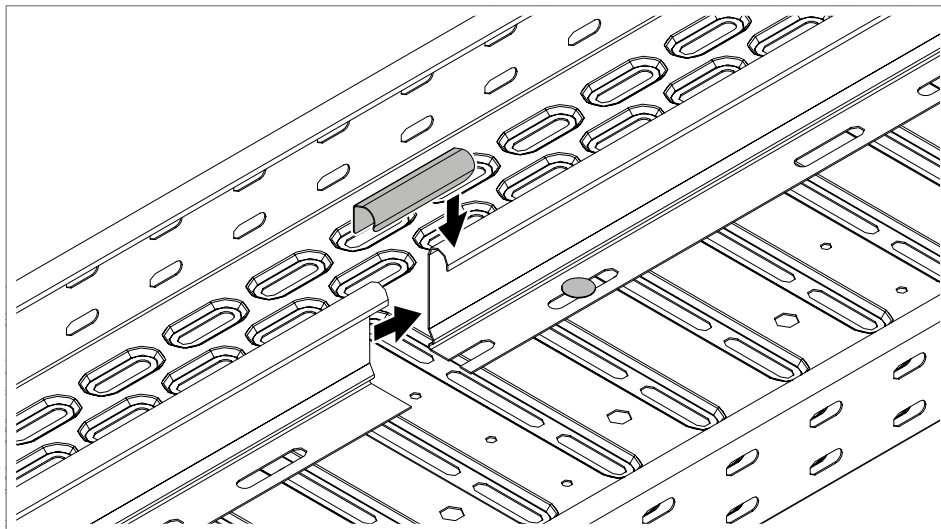
Slika 80: Spajanje pregrada
