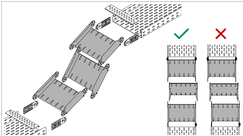
Slika 68: Element zglobne krivine sa polovinom zglobne spojnice i podnim završnim limom
