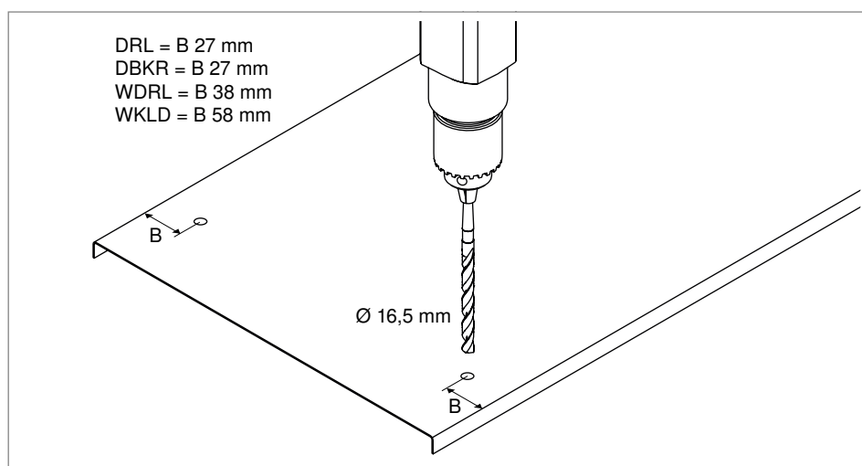
Slika 85: Prethodno bušenje poklopca
