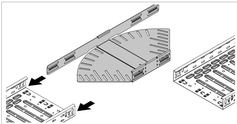
Slika 59: Ubacivanje krivine sa podesivim uglom
