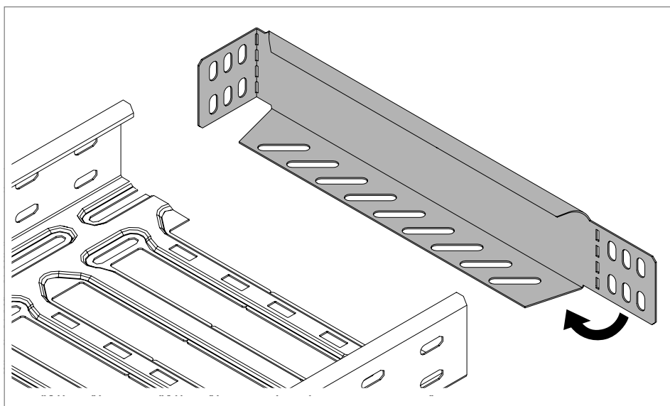
Slika 75: Savijanje jezička
