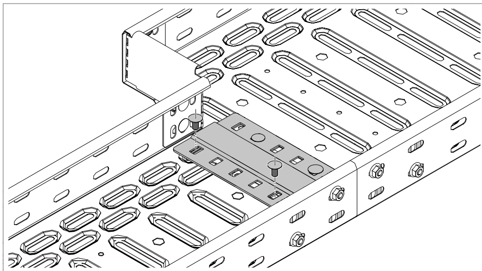
Slika 74: Učvrstiti prag zavrtnjima
