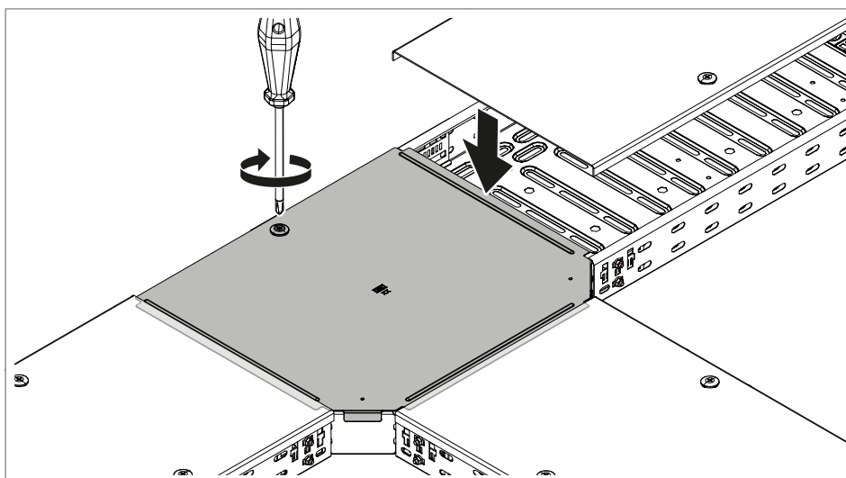
Slika 90: Osiguranje poklopca fazonskog komada sa poklopcem segmenta
