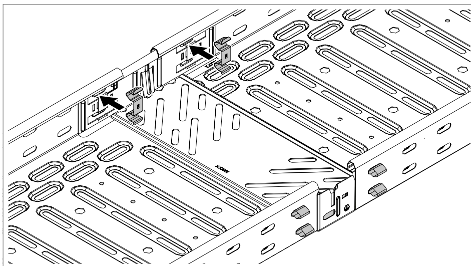
Slika 23: Fiksirati spojnicu dvostrukom stezaljkom
