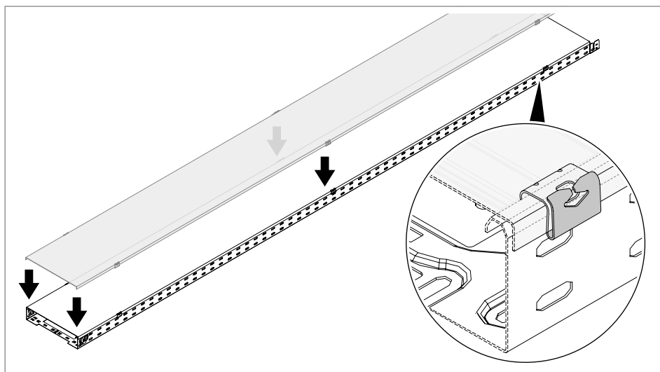
Slika 84: Uglavljivanje poklopca na mesto
