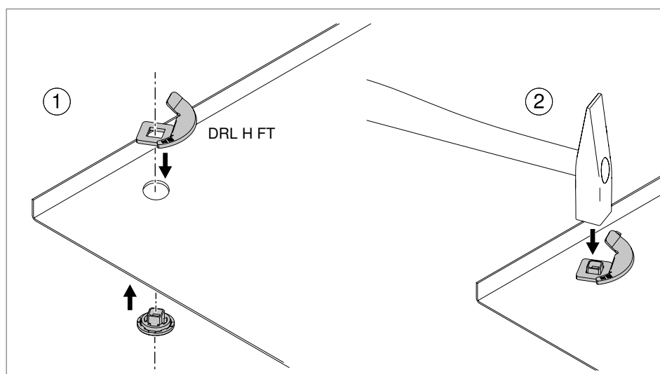
Slika 87: Učvršćivanje obrtne brave zakovicom
