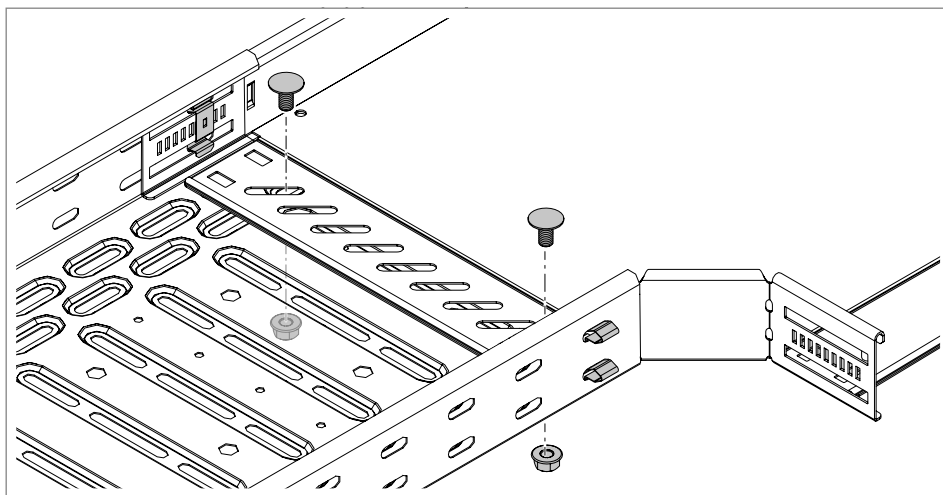
Slika 51: Učvrstiti prag zavrtnjima
