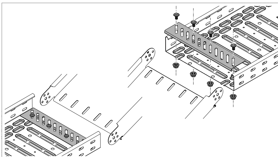
Slika 69: Montaža podnog završnog lima
