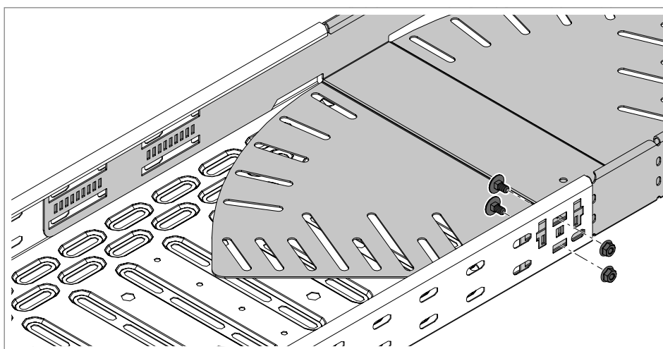
Slika 60: Fiksiranje krivine sa podesivim uglom
