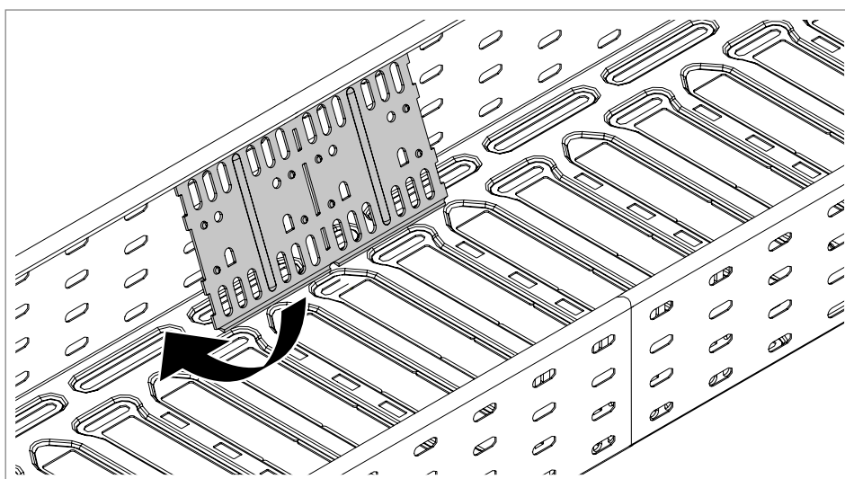
Slika 27: Postavljanje brze spojnice RLVL
