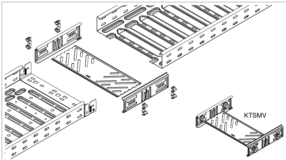
Slika 20: Brza spojica KTSM
