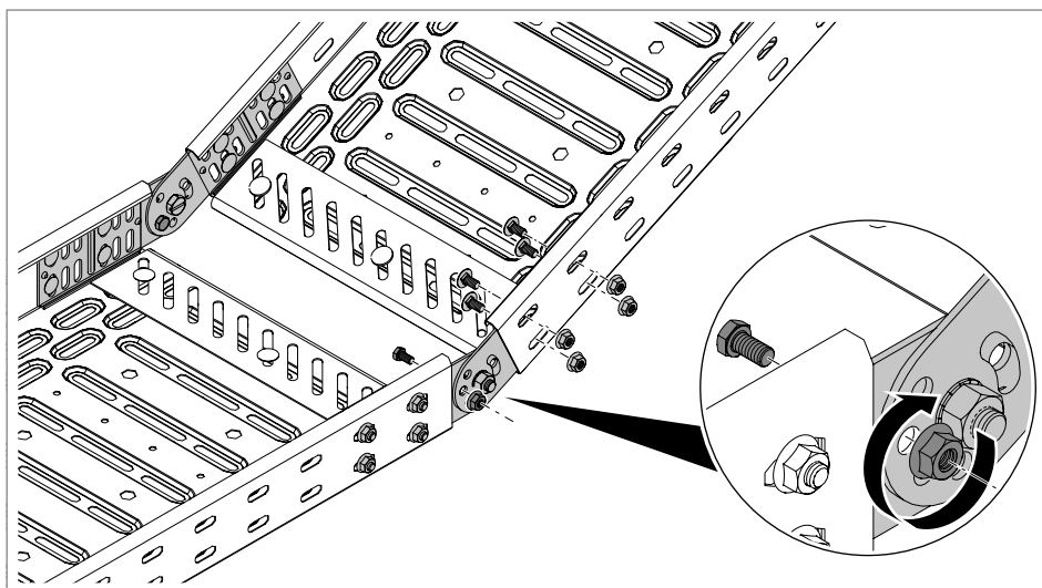
Slika 41: Zatezanje sigurnosnog zavrtnja
