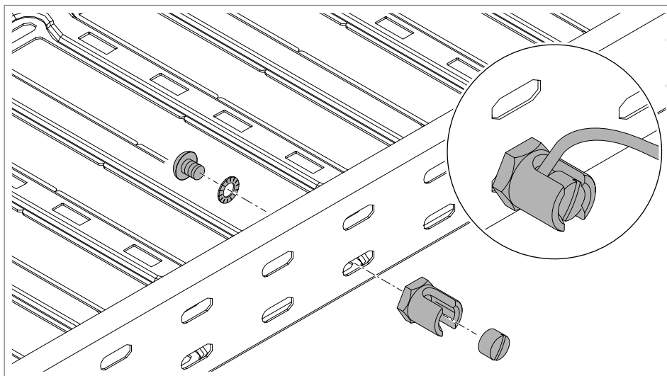
Slika 81: Montaža stezaljke za uzemljenje
