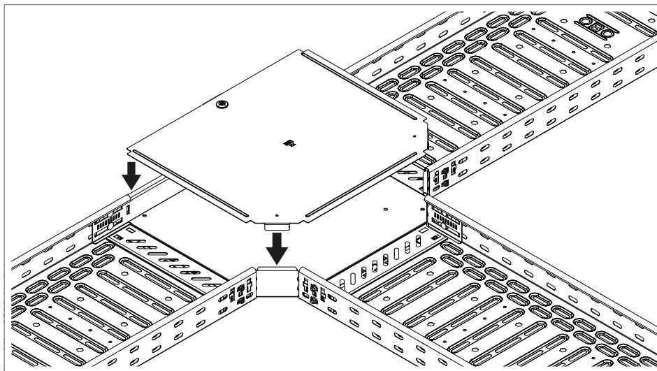
Slika 89: Postavljanje poklopca fazonskog komada
