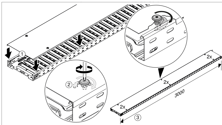
Slika 88: Montaža poklopca sa Helix obrtnom bravom
