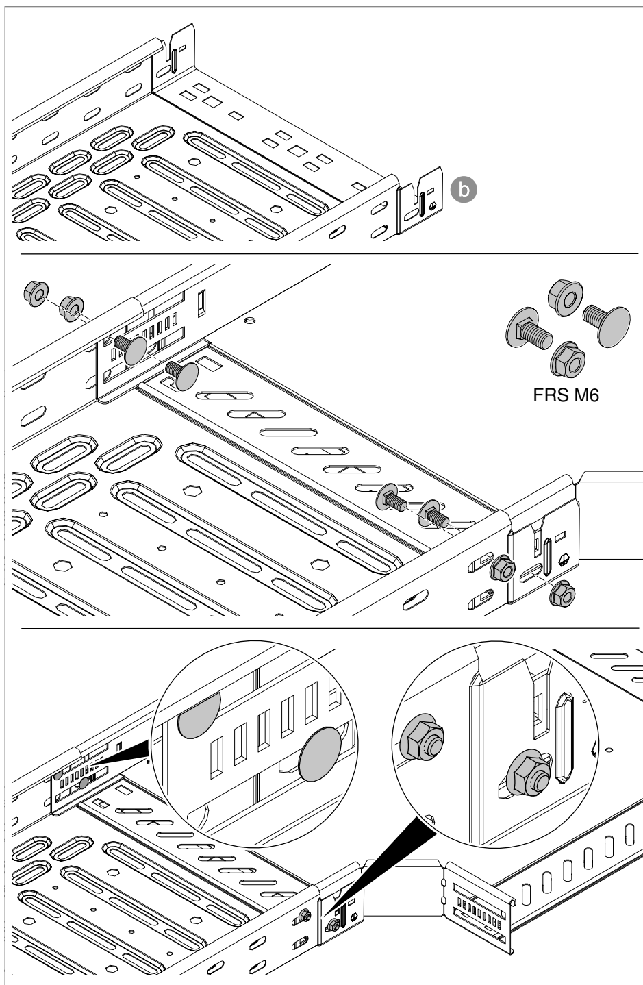
Slika 48: Učvršćivanje faznskog komada zavrtnjima (nerezani nosač kablova b)
