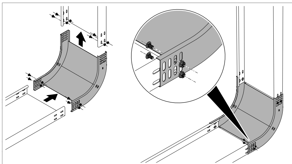
Slika 67: Montaža vertikalne krivine sa uzlaznim nagibom
