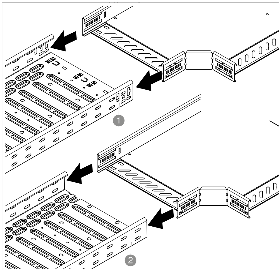
Slika 44: Umetanje fazonskog komada
