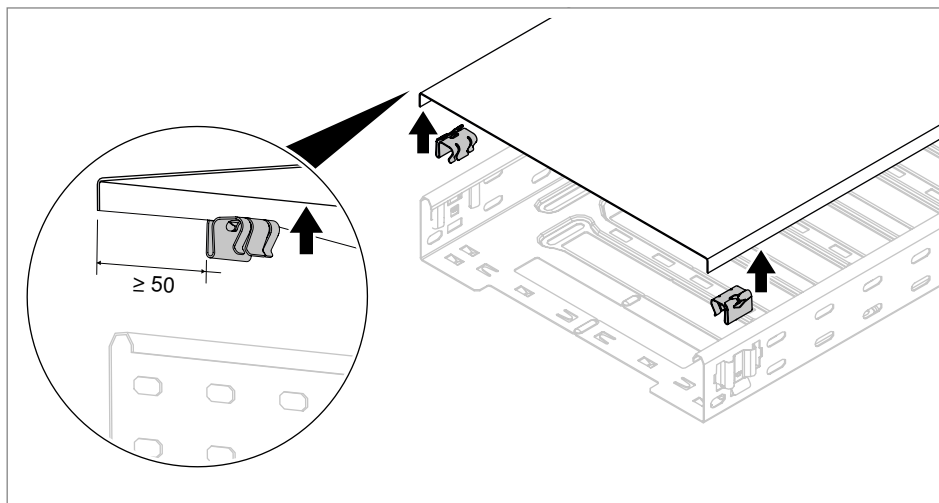
Slika 82: Postavljanje stezaljke poklopca na poklopac
