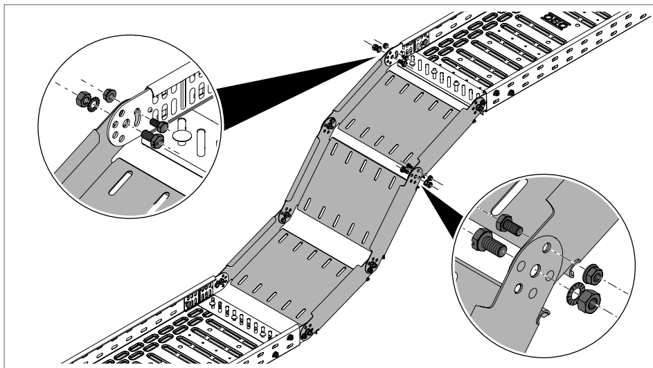
Slika 71: Montaža elemenata zglobnih podova
