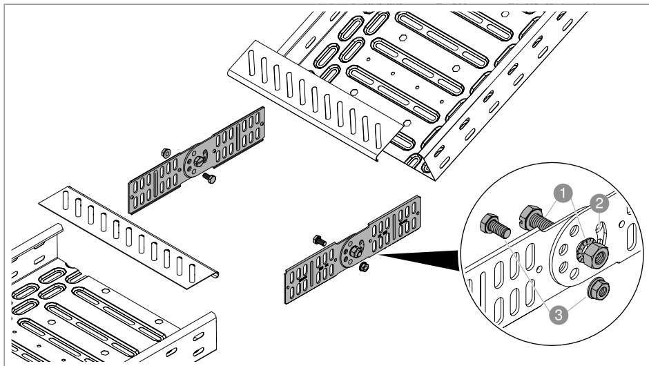
Slika 37: Zglobna spojnica RGV i podni završni limovi
