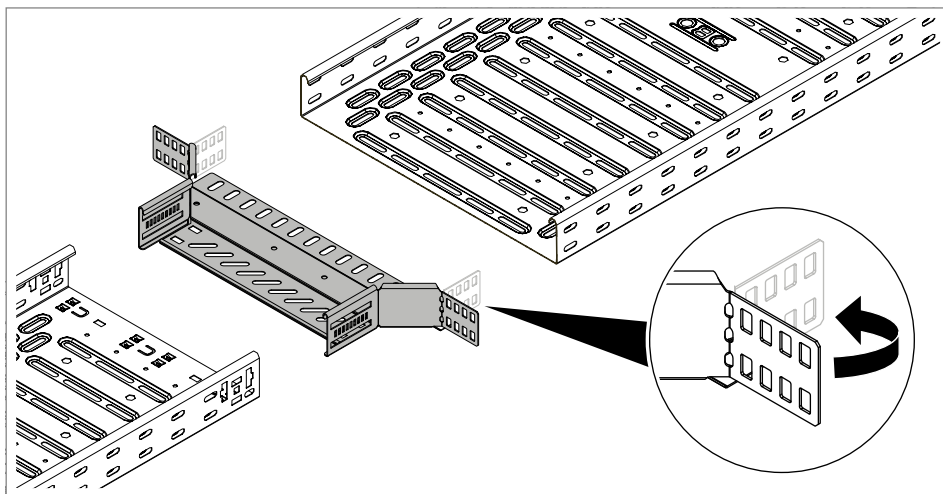
Slika 57: Savijanje jezička za spajanje
