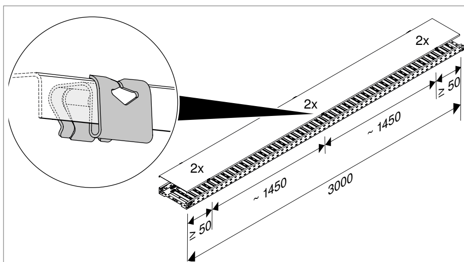
Slika 83: Raspoređivanje neophodnog broja stezaljki poklopca
