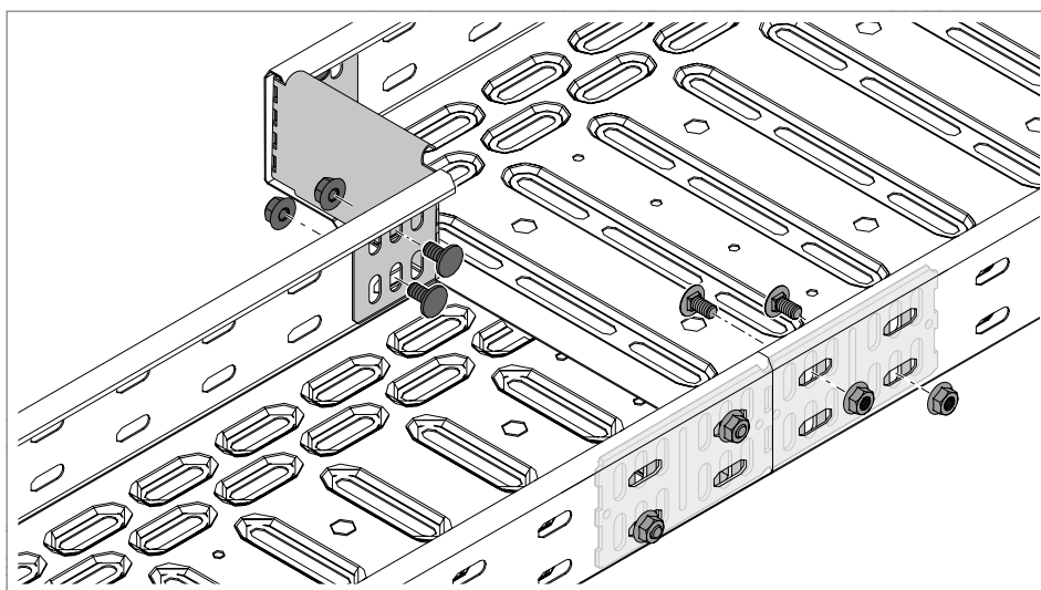
Slika 73: Montaža brze i ugaone spojnice i reducira
