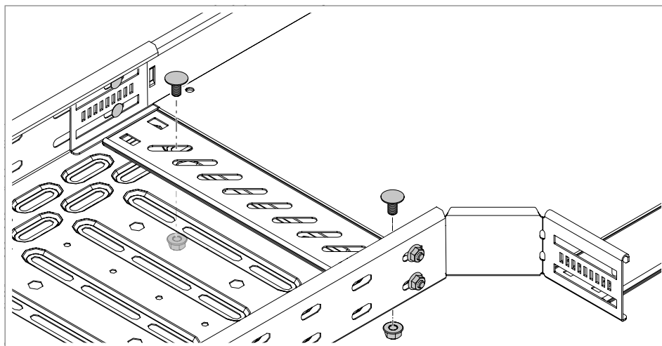
Slika 53: Učvrstiti prag zavrtnjima
