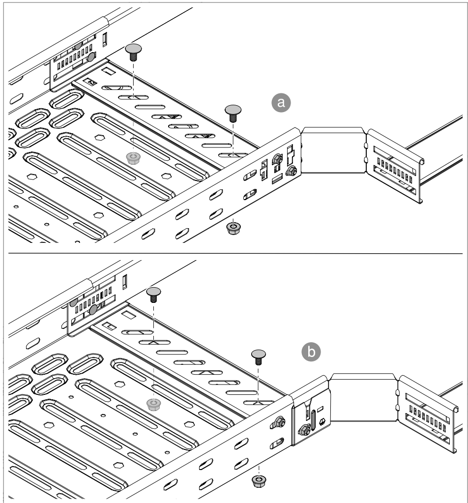
Slika 49: Učvrstiti prag zavrtnjima (nerezani nosač kablova a i b )
