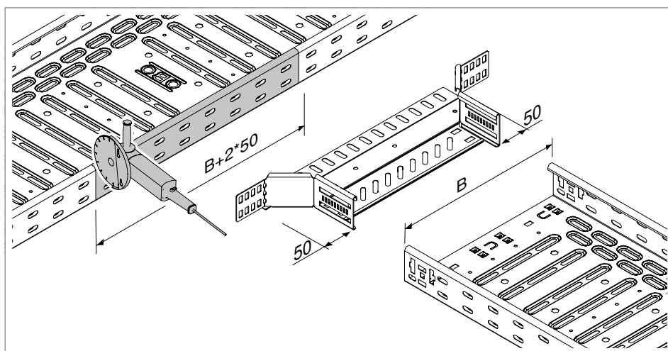
Slika 54: Izrezivanje bočne strane nosača kabla
