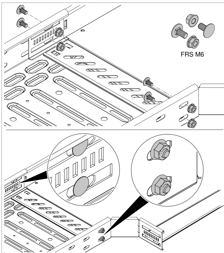
Slika 52: Učvršćivanje sa dvostrukim stezaljkama
