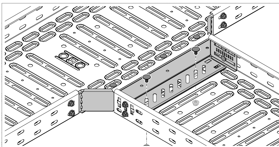
Slika 56: Učvršćivanje zavrtnjima nosača kablova za grananje na ugradnu račvu
