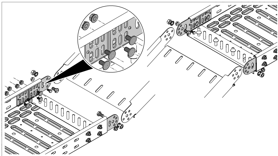
Slika 70: Montaža zglobne spojnice na nosače kablova
