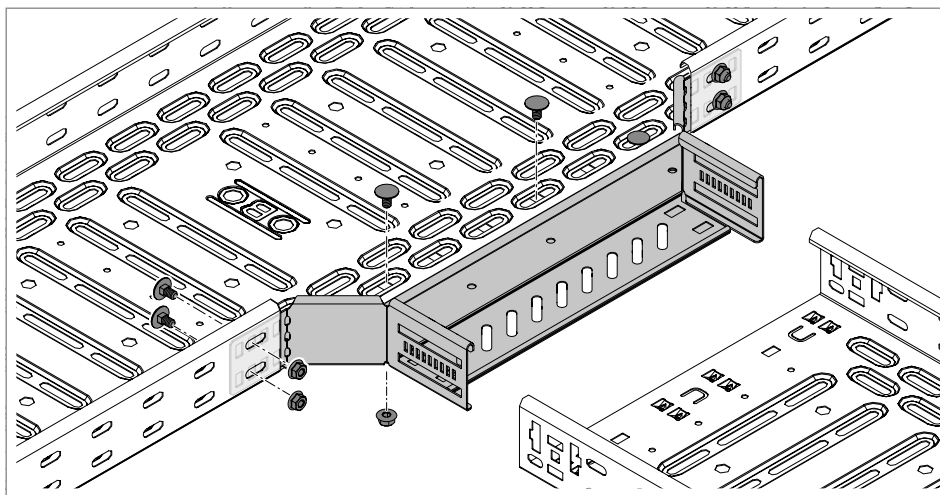
Slika 55: Učvršćivanje ugradne račve na neprekidni nosač kablova
