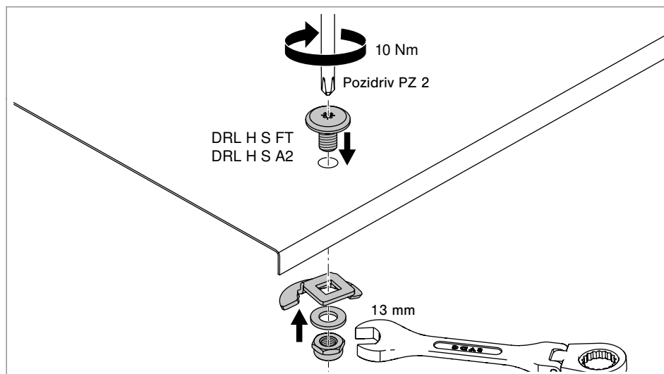
Slika 86: Učvršćivanje obrtne brave zavrtanjima
